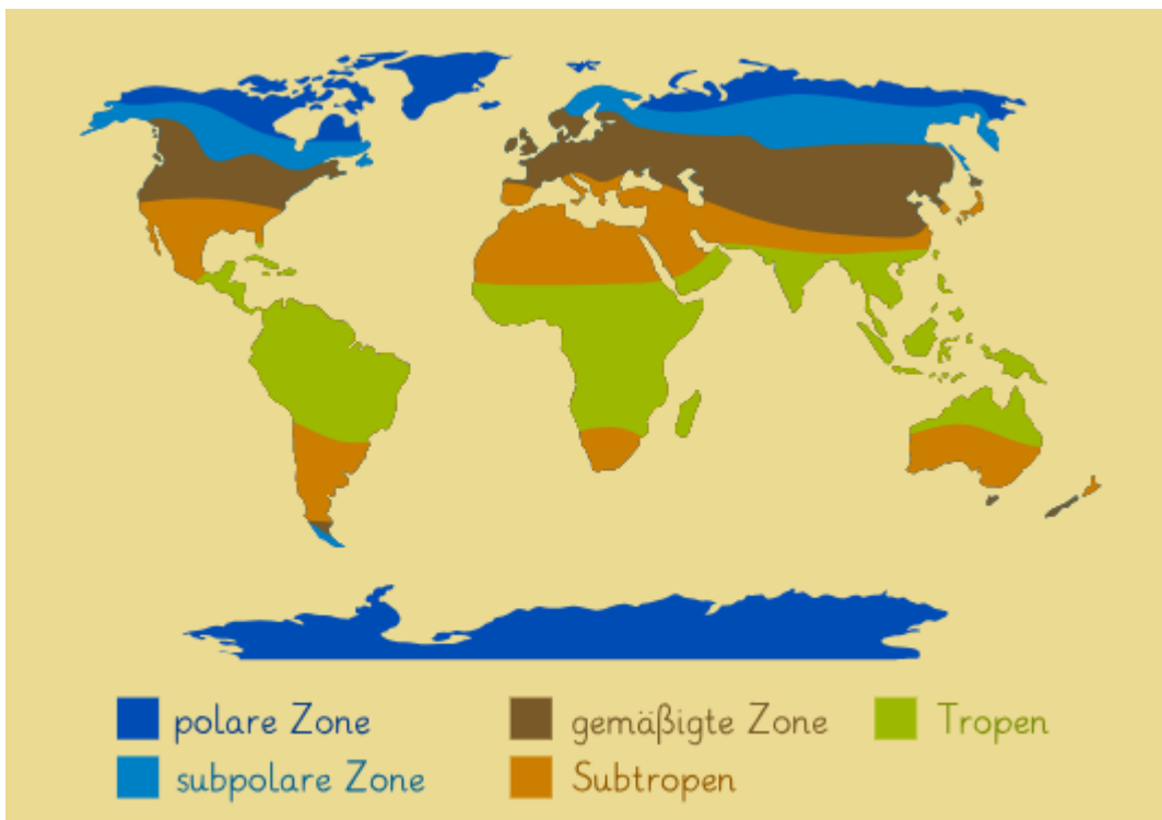
Klimazonen der Erde (vereinfacht)
