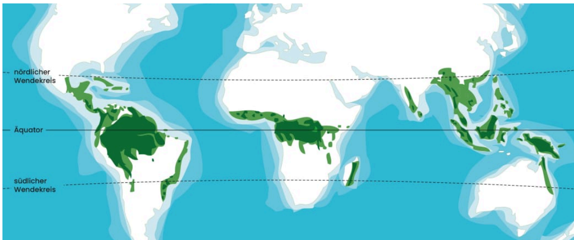
die Verbreitung der tropischen Regenwälder auf der Erde
