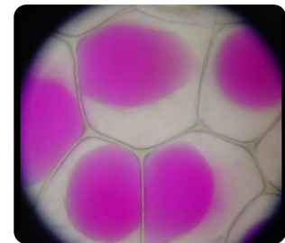
Plasmolyse
