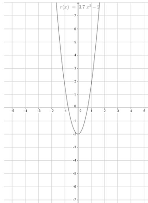
(6) r(x) = 3.7x^2 - 2
