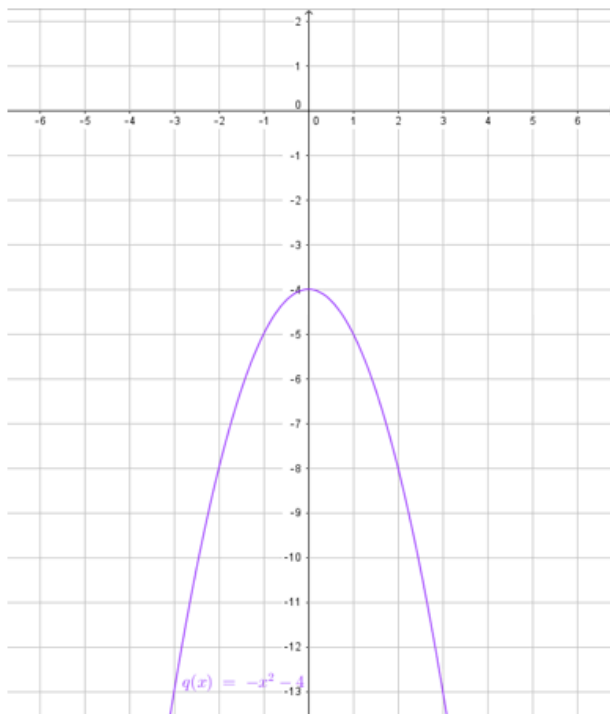
(5) q(x) = -x^2 - 4
