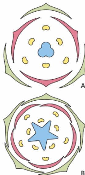
2 Blütendiagramme
