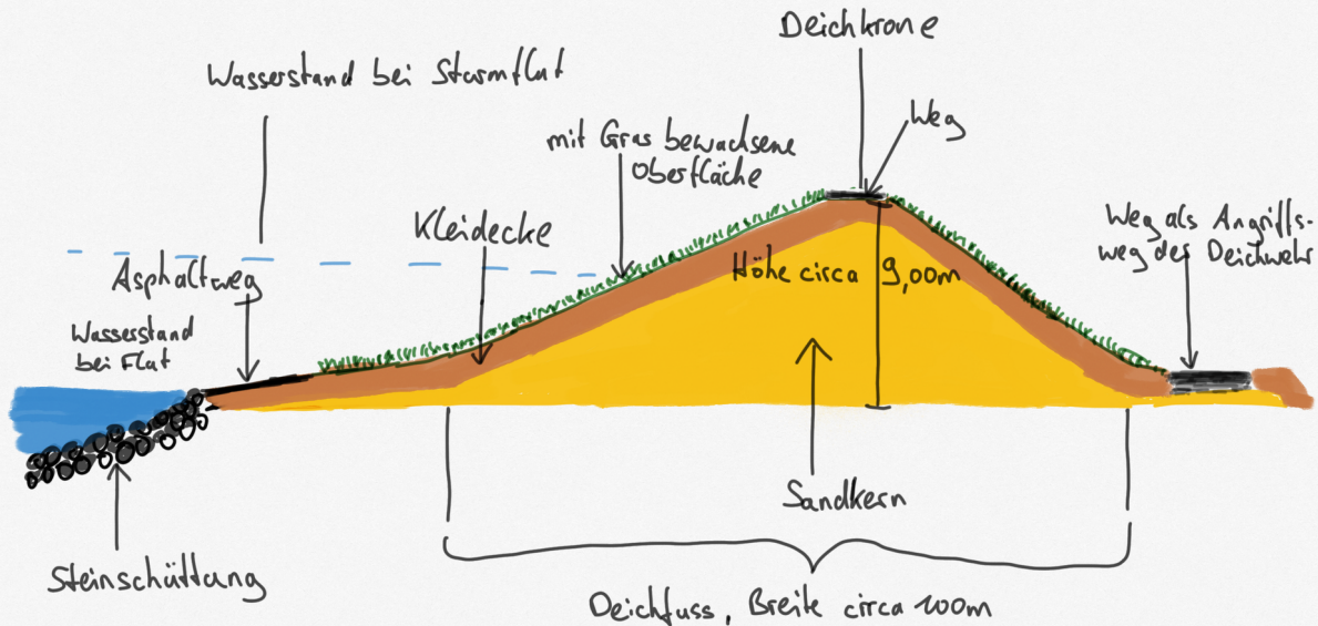
Deichquerschnitt
