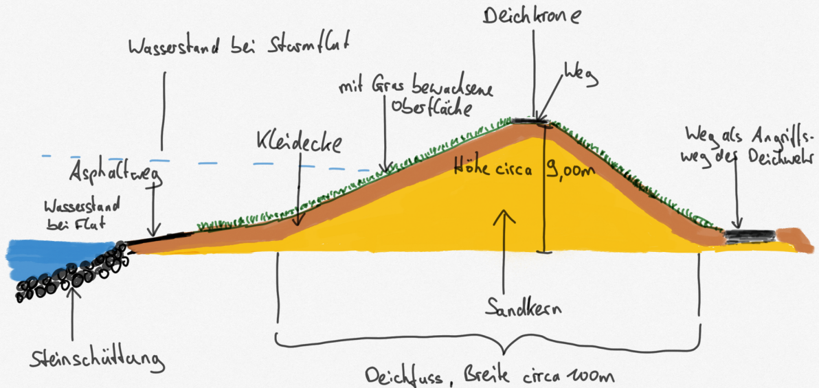
Deichquerschnitt
