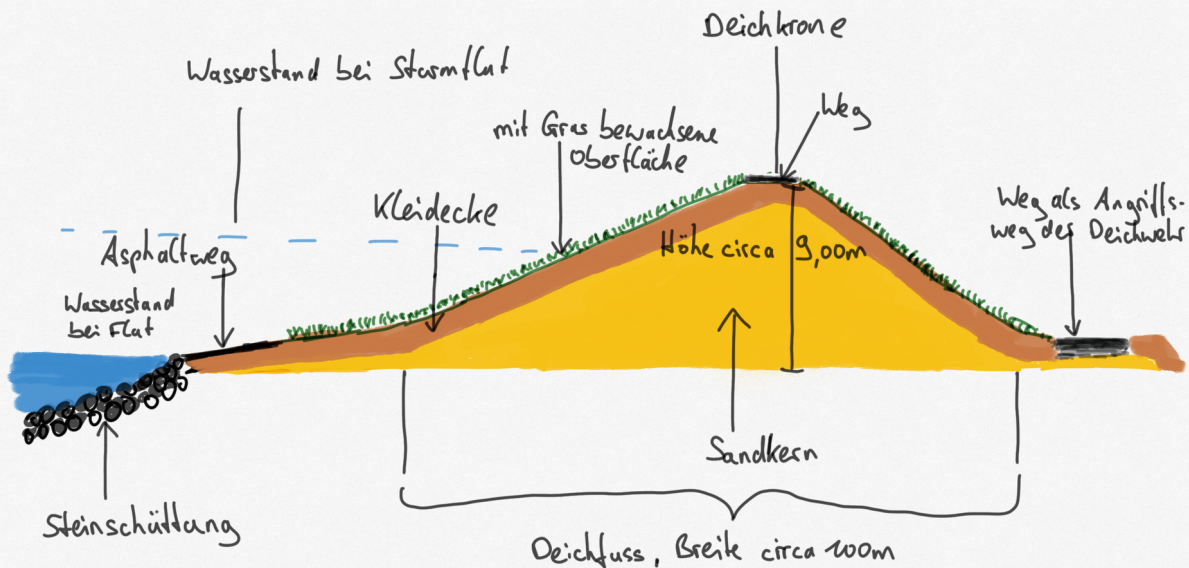
Deichquerschnitt
