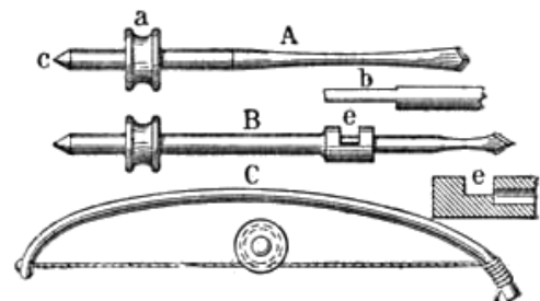
Bogen und Bohrer
