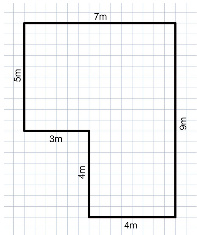
Grundriss des Unterstandes
